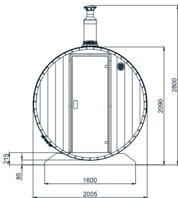
čelní pohled
