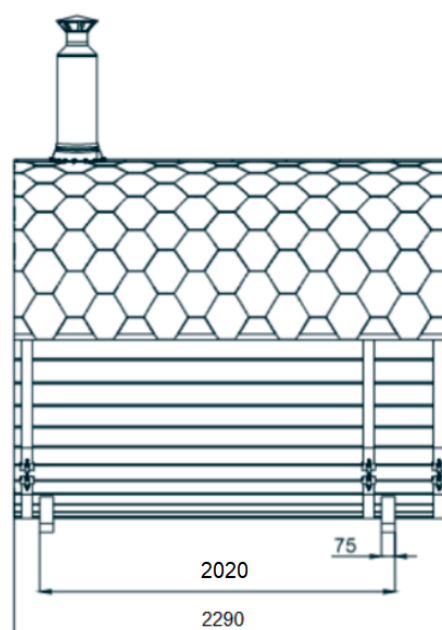
boční pohled
